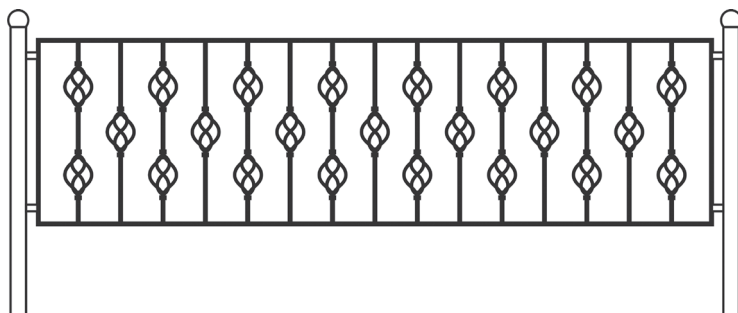
Ог-08 □ 20x20 ∅12 ≧ 18x2 Элемент №159/3 (504/6)
