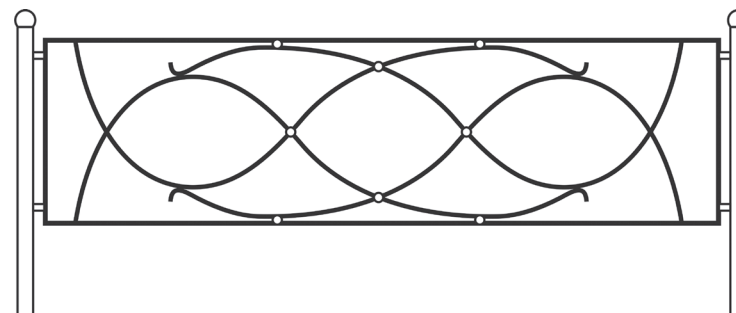
Ог-12 □ 20x20 ∅12 Элемент №882/30
