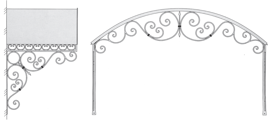
К-004 □ 40x20 □ 20x20 ∅ 10 ∅ 12 Лист. 1 ≡ 40x4 ≡ 18x2
